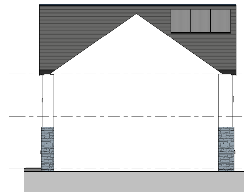
ADJOINING SIDE ELEVATION 1 : 100 PLOT 6 + 7
